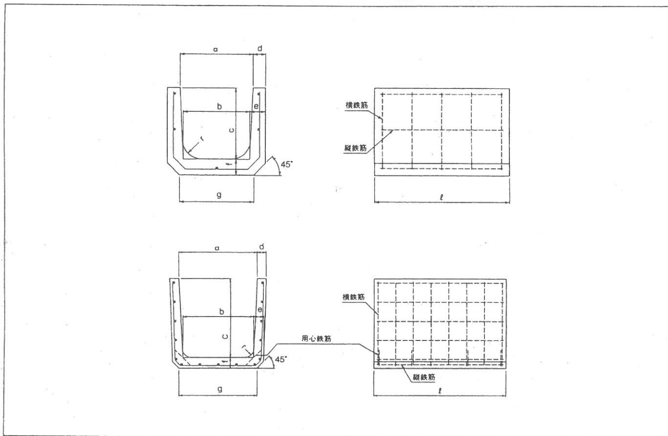
寸法・配筋・質量表
