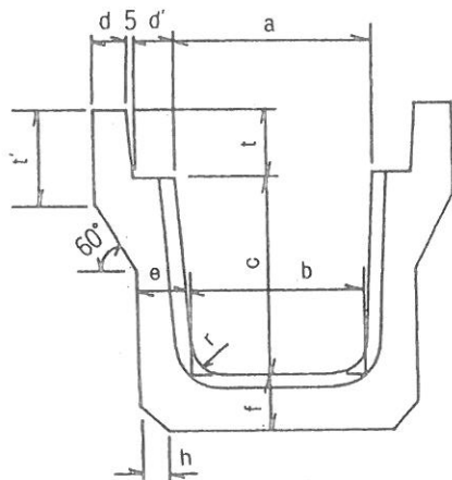
目地部(参考図)
