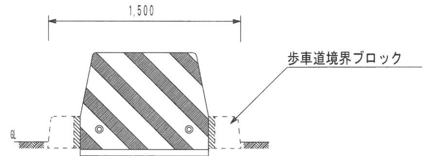
背面図
