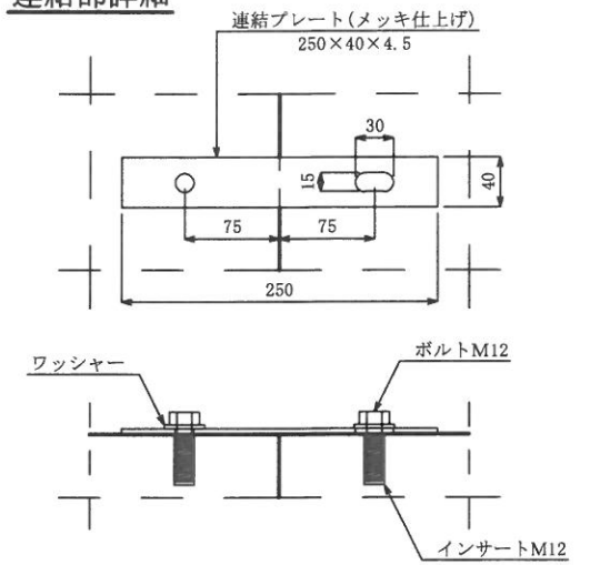
連結部詳細
