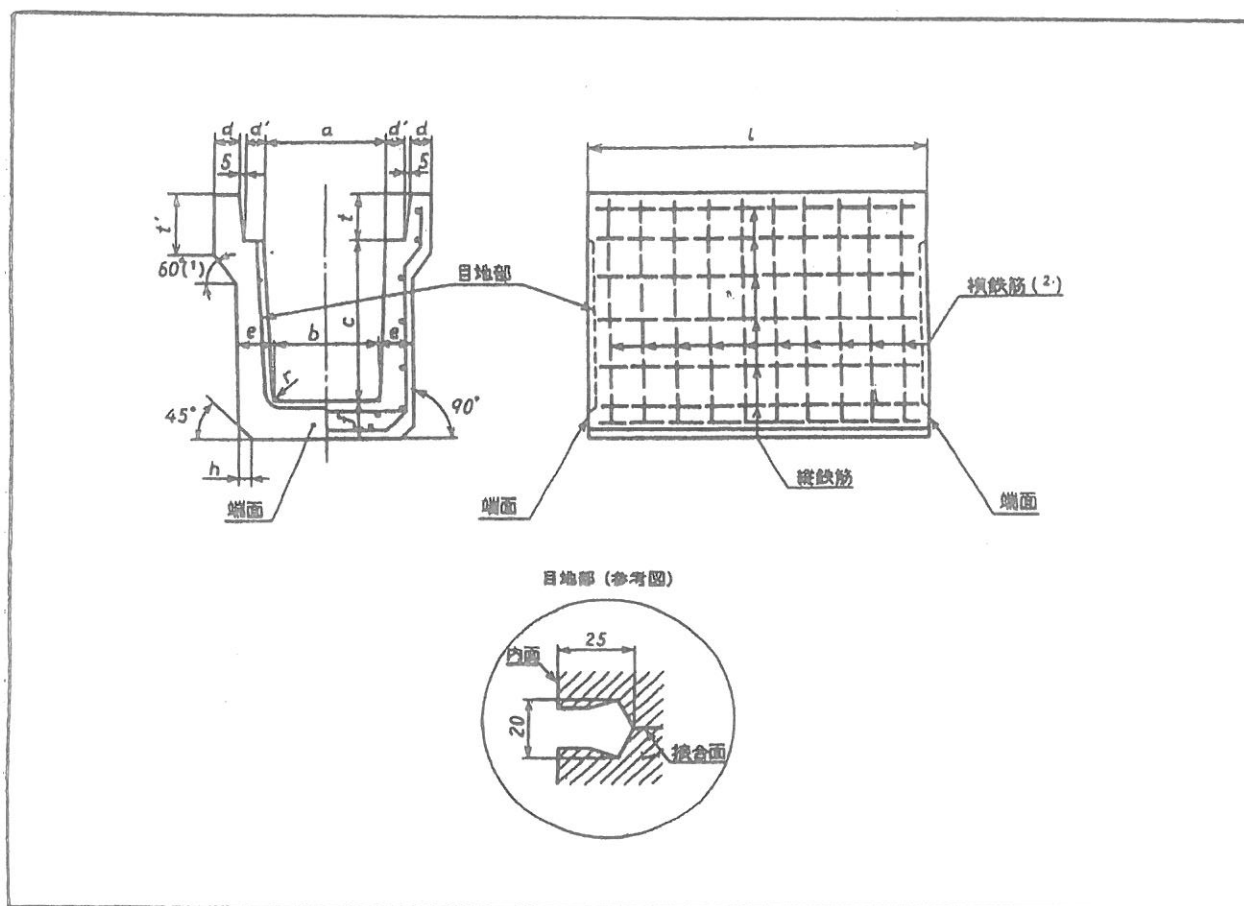
寸法・配筋・質量表
